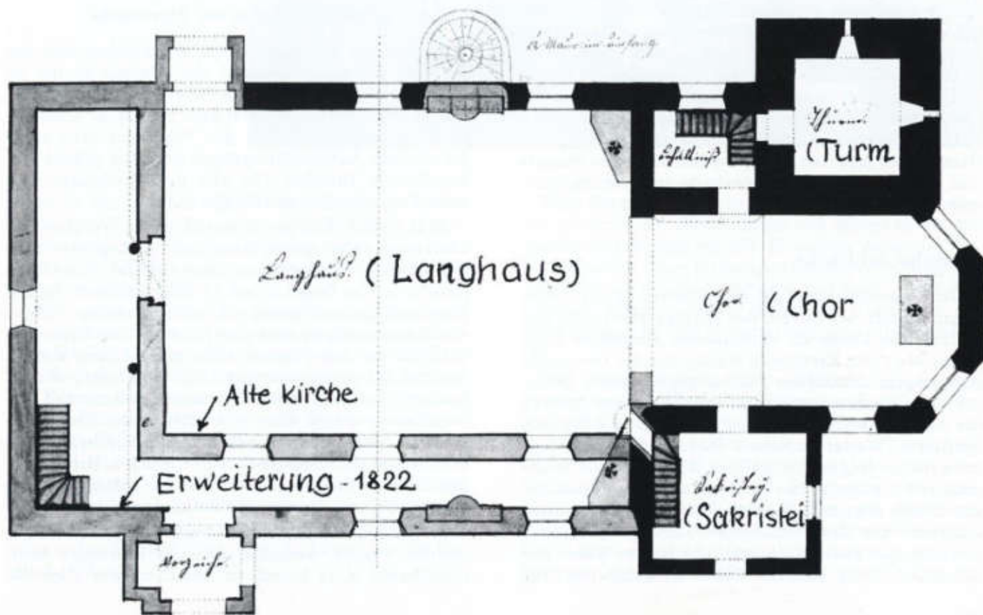
Grundriß der Pfarrkirche St. Michael – von Maurermeister Köpfle, Landsberg – 1822
